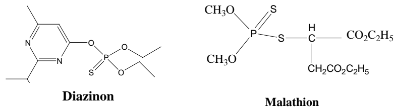
Gambar 4. Struktur organofosfat
